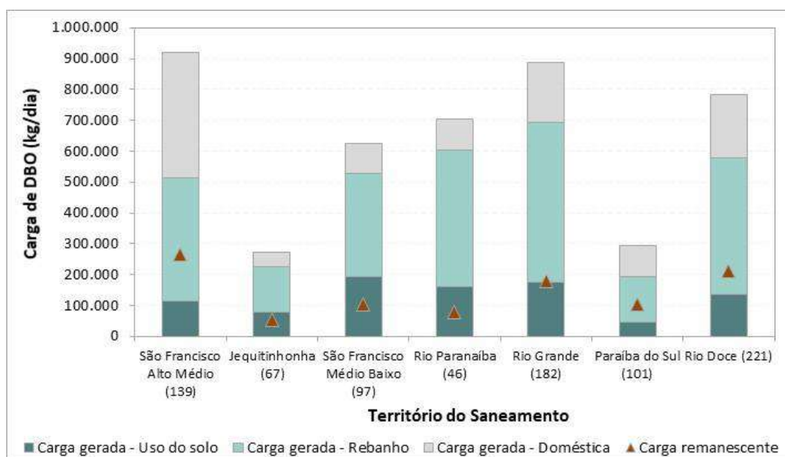
Figura 5.84 – Cargas de DBO por fonte e Território do Saneamento
