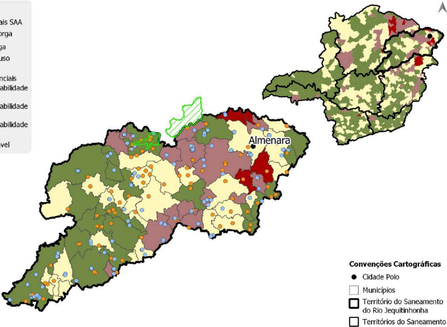
Figura 5.32 – Distribuição das captações de SAA no TS-2 segundo outorga, vulnerabilidade quantitativa da sede municipal e áreas de conflito pelo uso dos recursos hídricos
