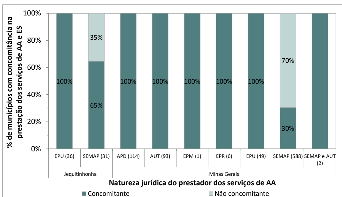
Figura 5.71 – Concomitância na prestação dos serviços de abastecimento de água e esgotamento sanitário no TS-2 e em Minas Gerais, em relação a natureza jurídica do prestador dos serviços de abastecimento de água nas sedes municipais
