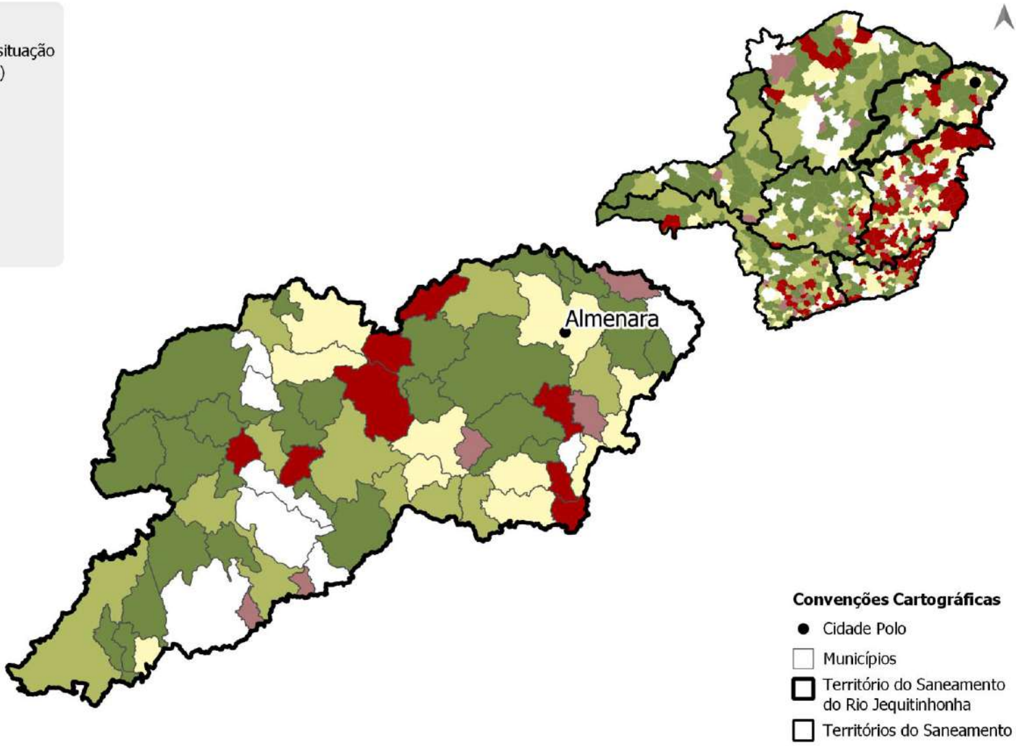
Figura 5.147 – Parcela de domicílios em situação de risco de inundação
