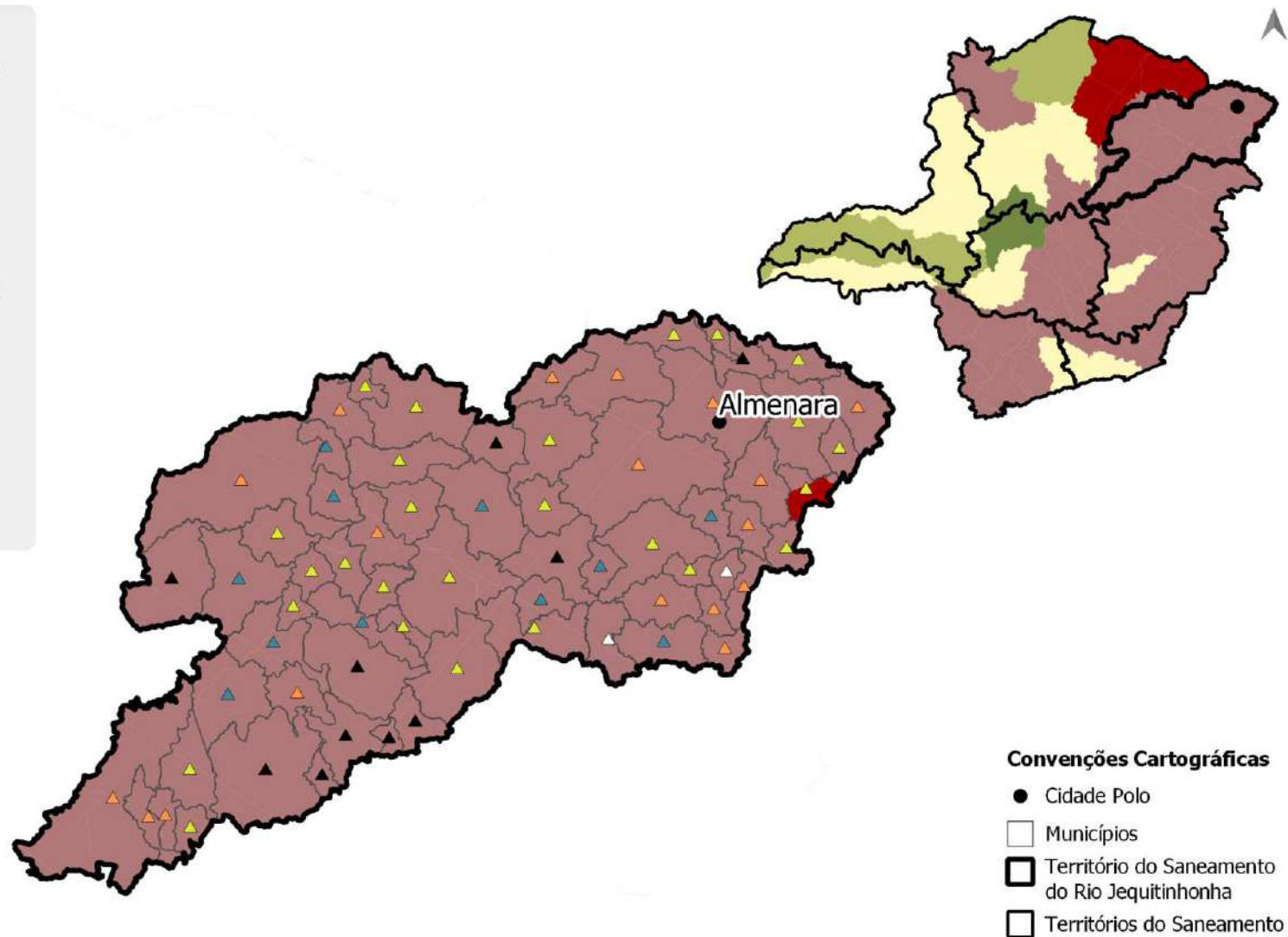
Figura 5.4 – Vulnerabilidade natural à disponibilidade hídrica subterrânea e vulnerabilidade climática
