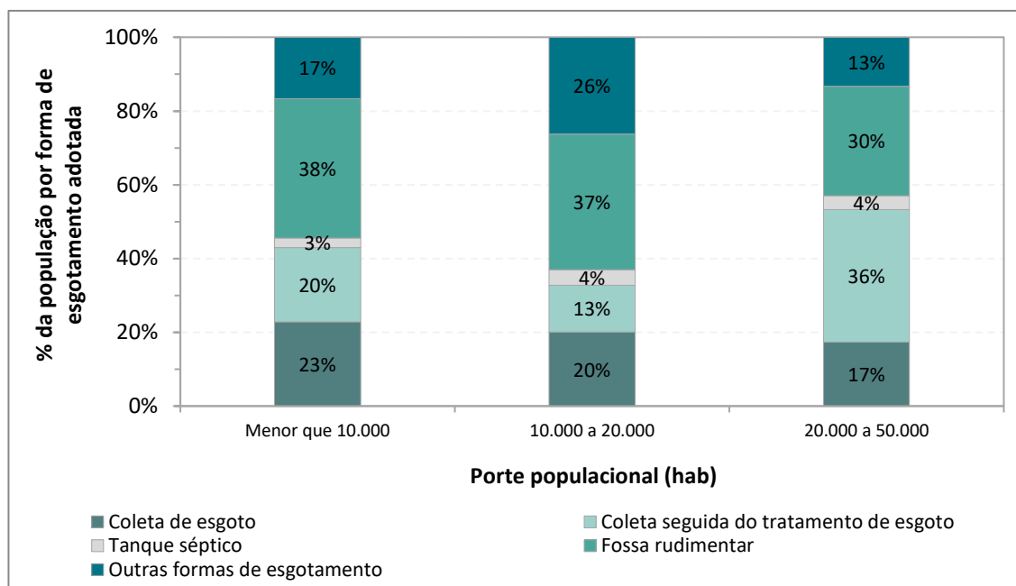
Figura 5.76 – Percentual de população e formas de afastamento (e tratamento) do esgoto adotadas por porte populacional
