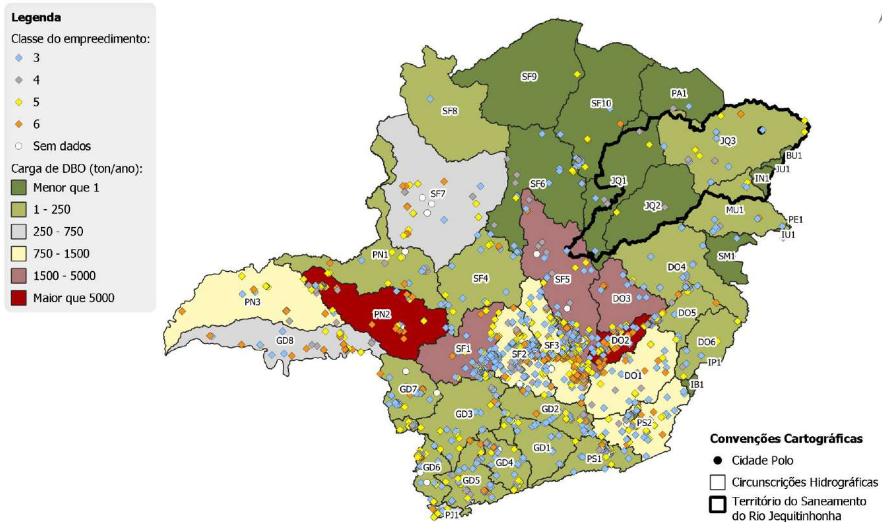
Figura 5.88 – Somatório da carga remanescente de DBO nas CH e classes dos empreendimentos
