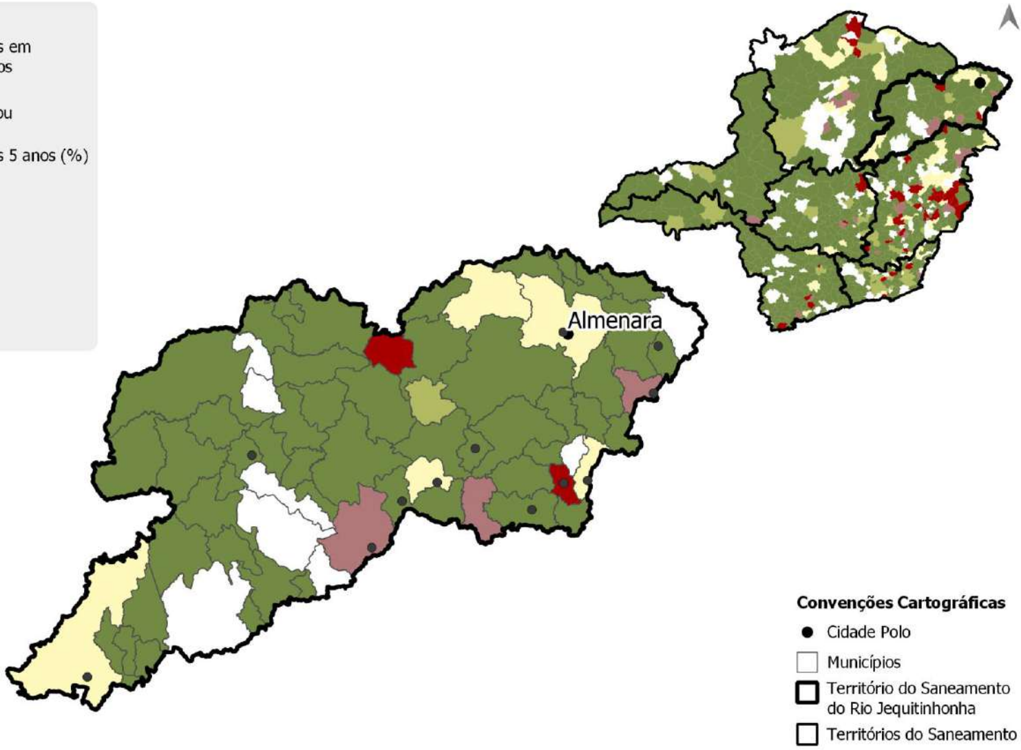
Figura 5.148 – Parcela de desabrigados por eventos pluviométricos nos municípios do TS-2 (2013-2019)
