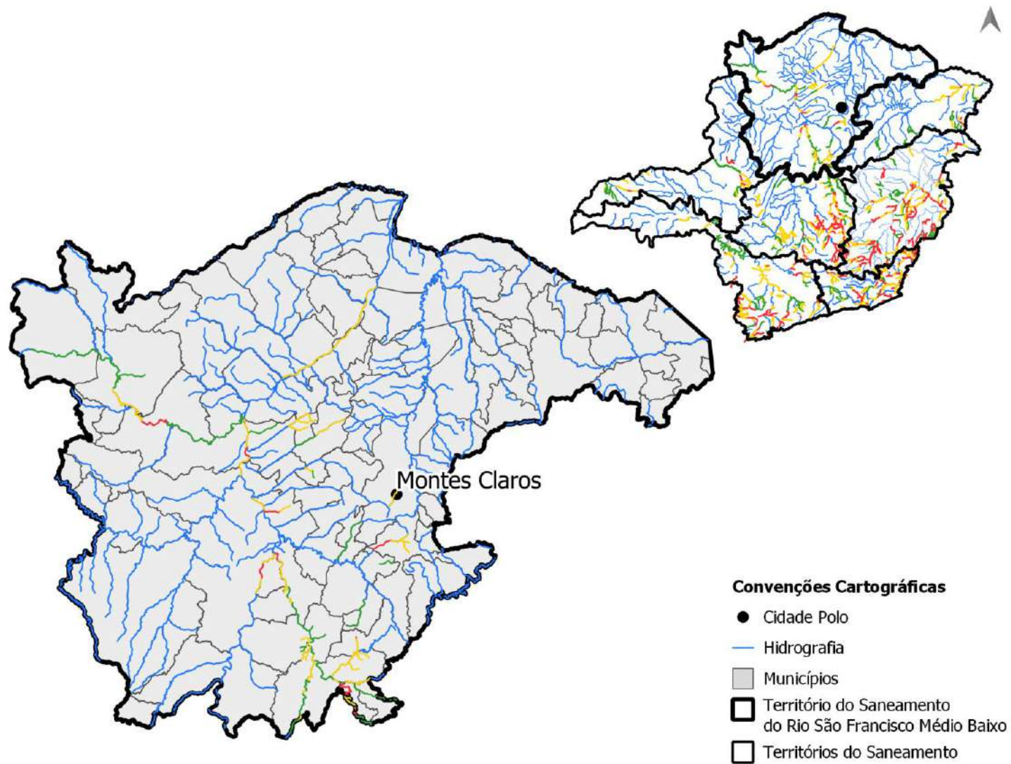
Figura 5.149 – Vulnerabilidade a inundações em cursos d’água do Território
