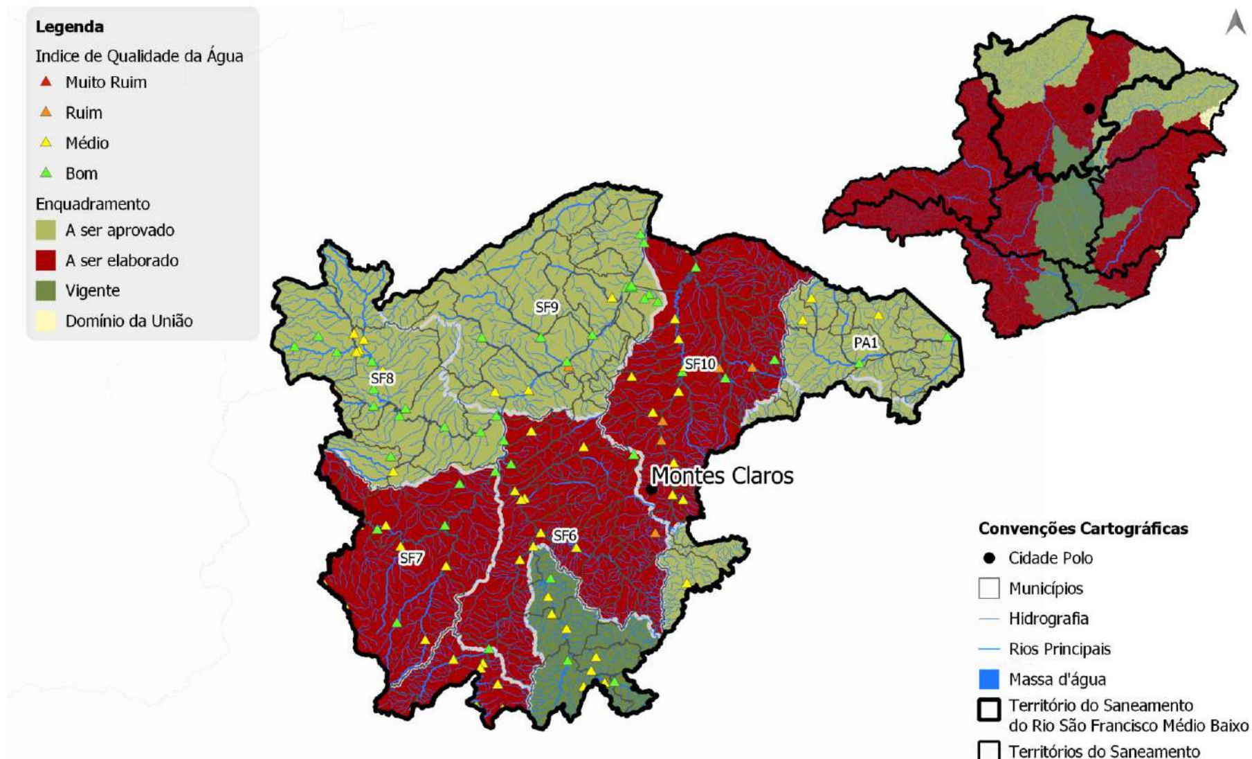
Figura 5.6 – Situação do enquadramento das bacias hidrográficas do TS-3 e índice de qualidade da água
