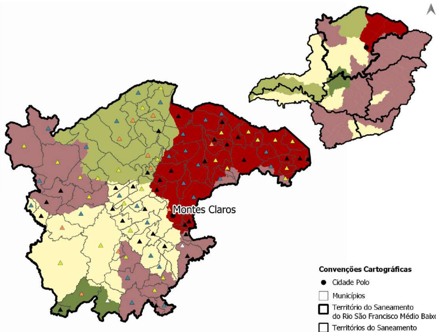
Figura 5.4 – Vulnerabilidade natural à disponibilidade hídrica subterrânea e vulnerabilidade climática
