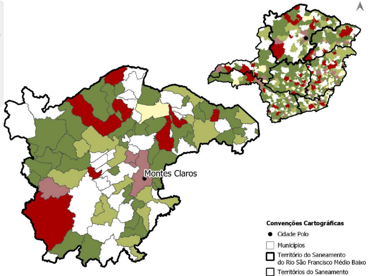
Figura 5.151 – Ocorrência de enxurradas, alagamentos e inundações no TS-3, no período entre 2015-2019
