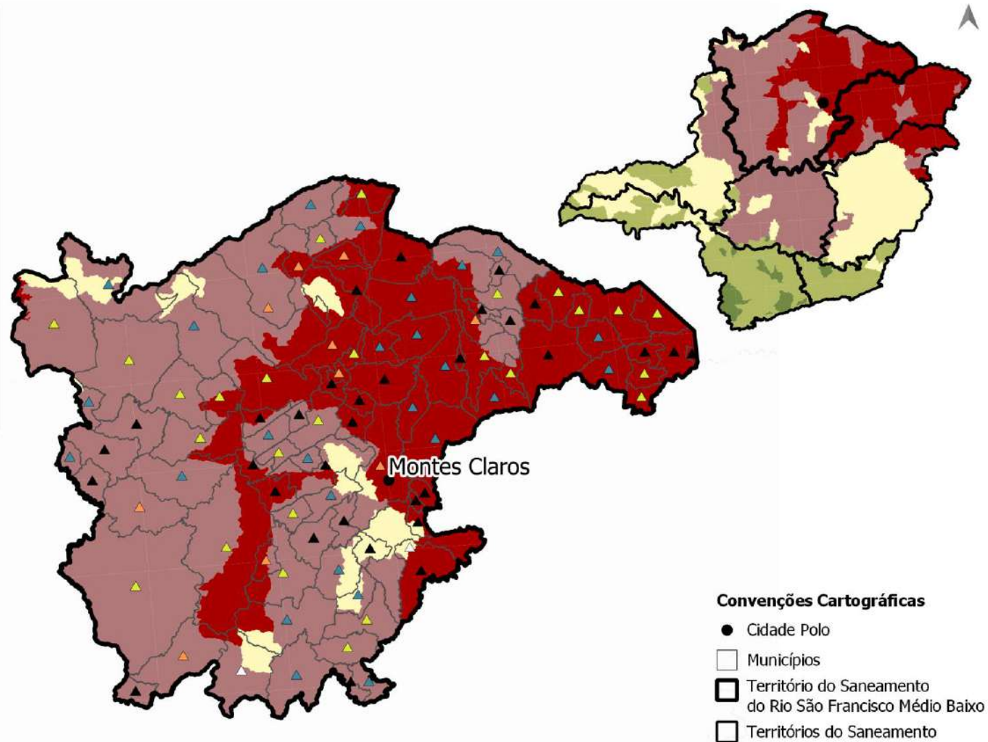
Figura 5.3 – Mapa de vulnerabilidade natural à disponibilidade hídrica superficial e vulnerabilidade climática
