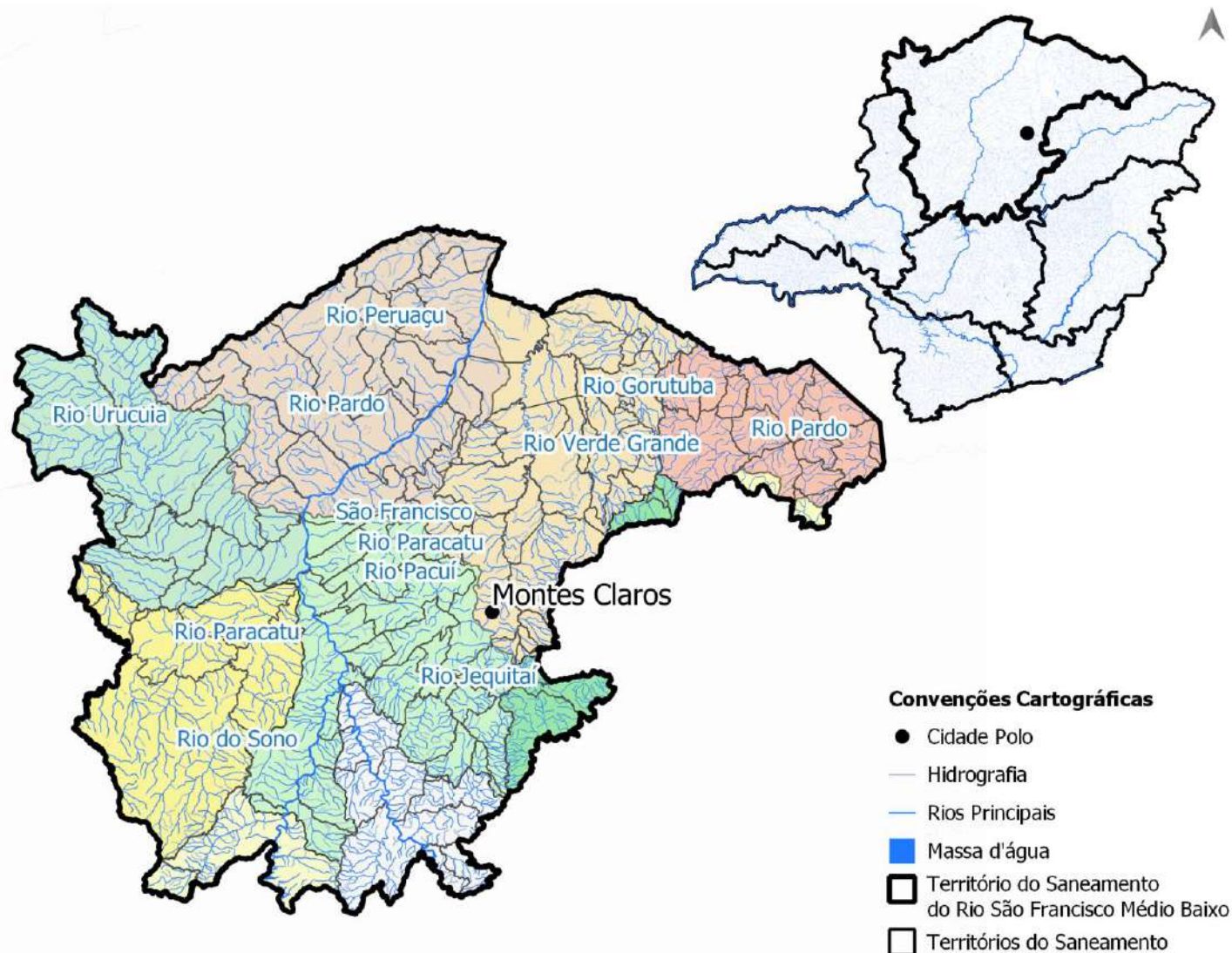
Figura 5.1 – Hidrografia superficial e circunscrições hidrográficas do TS-3
